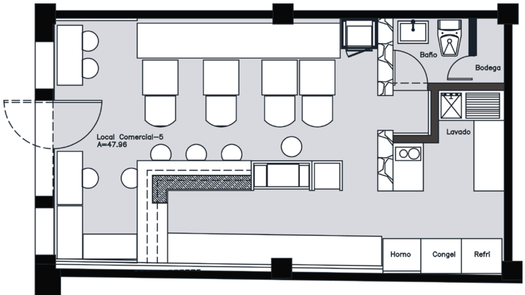
Nombre del proyecto: El Callejón Café. Diseño del proyecto: Boué Arquitectos / Arq. Gerardo Boué. Año: 2016 Ubicación: Ciudad de México. Construcción: 47 m 2 Fotografía: © Marcos Betanzos.
